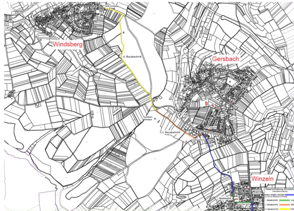
Trassenplanung Gas-Transport
